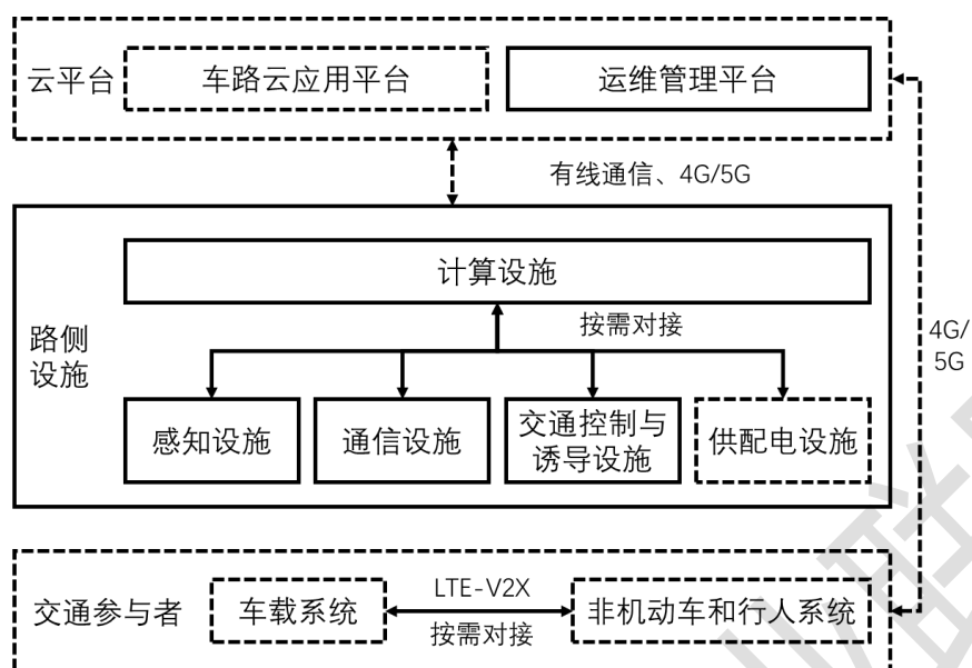
图1 路侧设施运维管理总体架构
