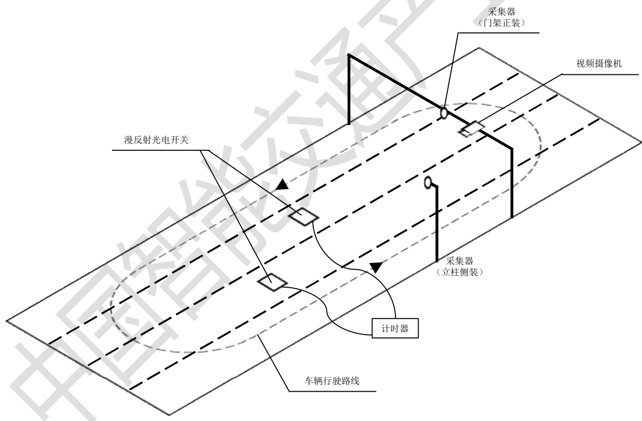
图B.1 试验场测试环境示意图
