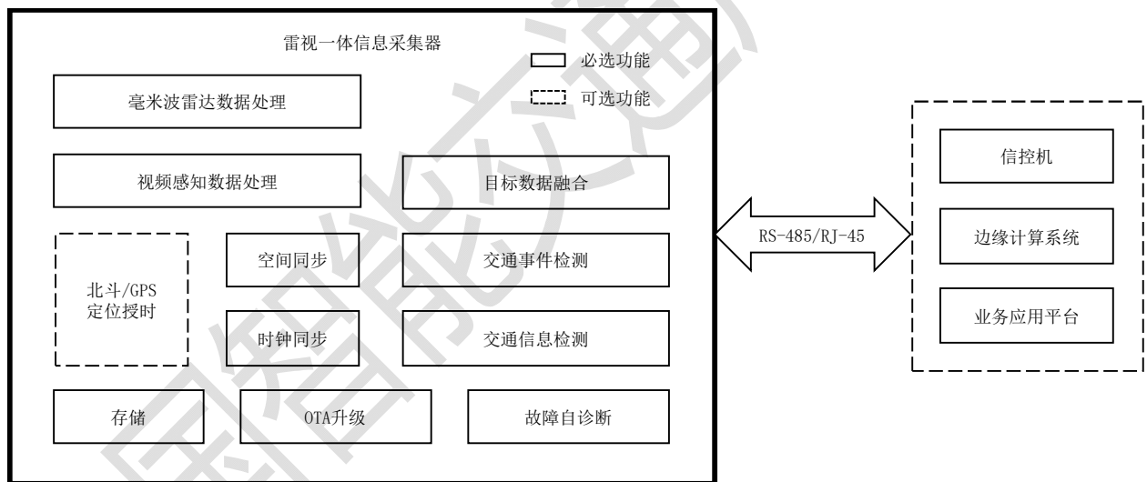
图1 采集器功能组成示意图
