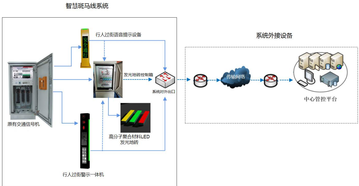
图 1 智慧斑马线系统拓扑图
