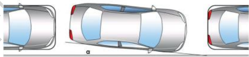
图 14 \alpha 的定义：车辆与路缘的方向角。在本例中为正向角
