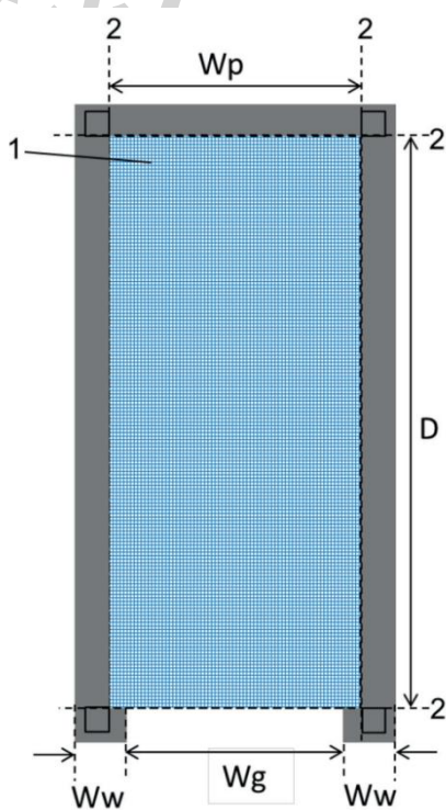
图 7 -车库门的几何形状
