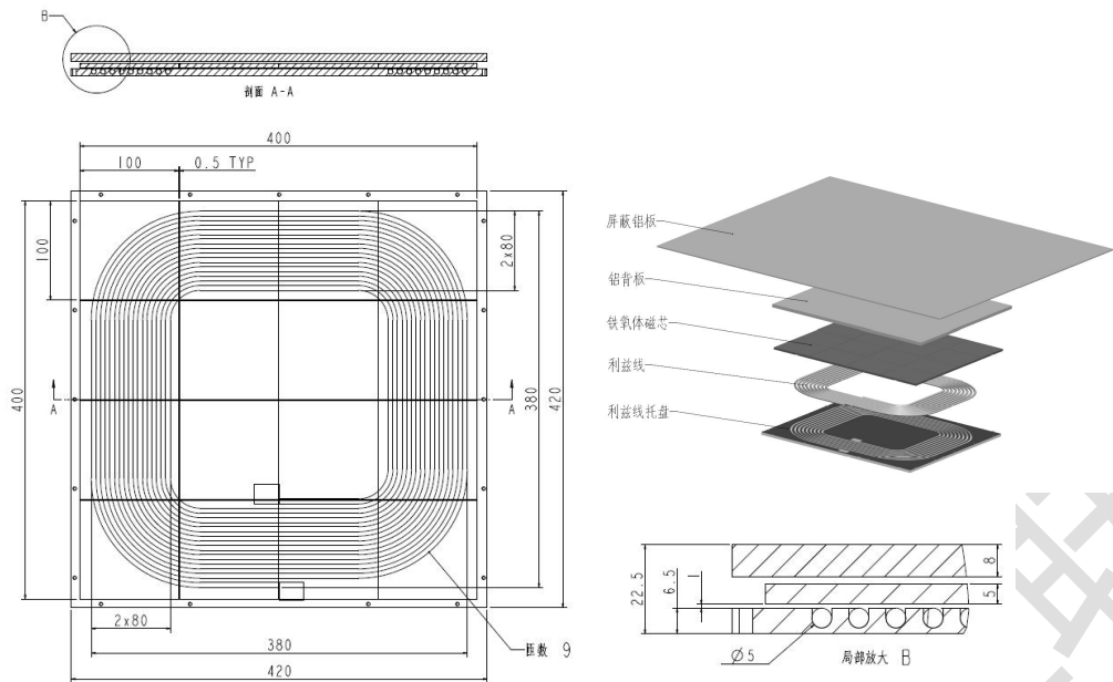
图 B.3 MF-WPT1 Z3 的车载参考设备的机械结构
