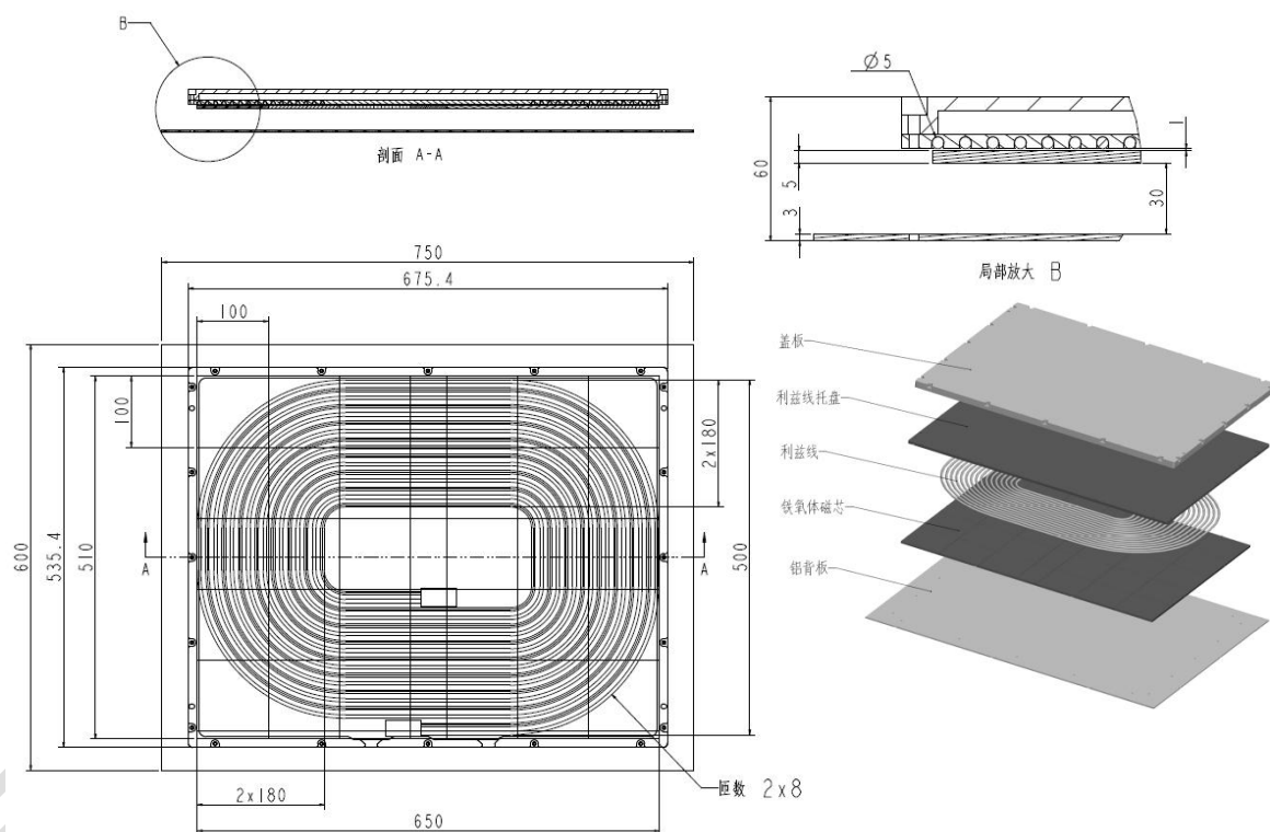
图 A.1 地面参考设备结构
