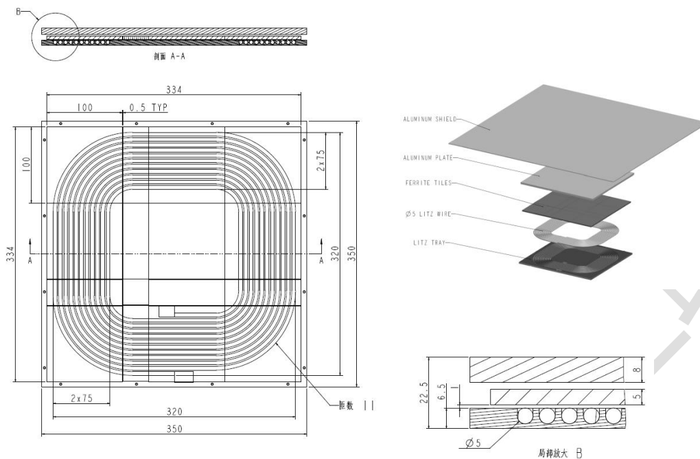
图 B.10 MF-WPT3 Z2 的车载参考设备的机械结构
