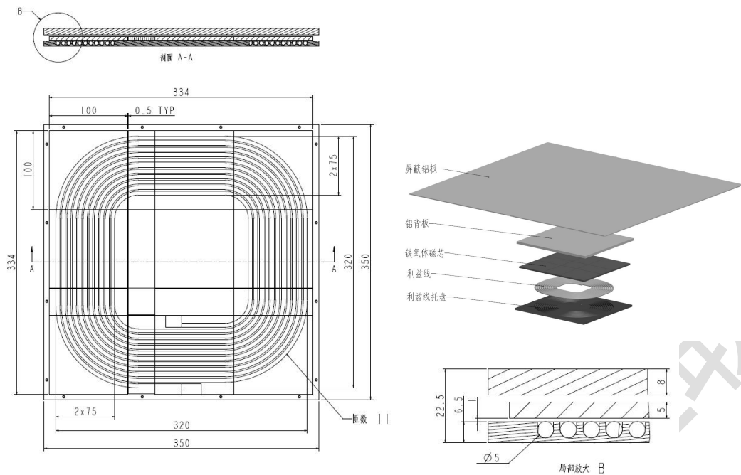
图 B.6 MF-WPT2 Z2 的车载参考设备的机械结构
