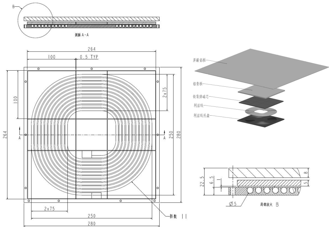
图 B.1 MF-WPT1 Z1 的车载参考设备的机械结构
