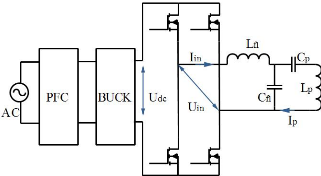
图 A.2 地面参考设备的主电路拓扑
