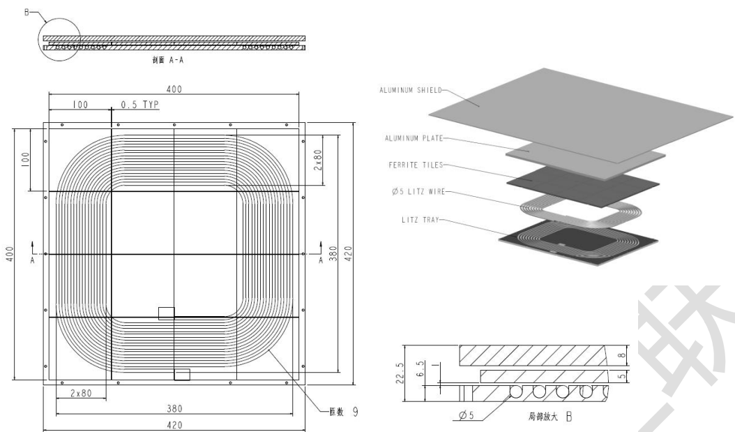
图 B.11 MF-WPT3 Z3 的车载参考设备的机械结构
