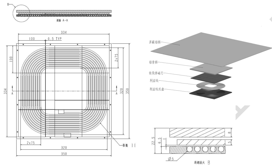
图 B. 2 MF-WPT1 Z2 的车载参考设备的机械结构
