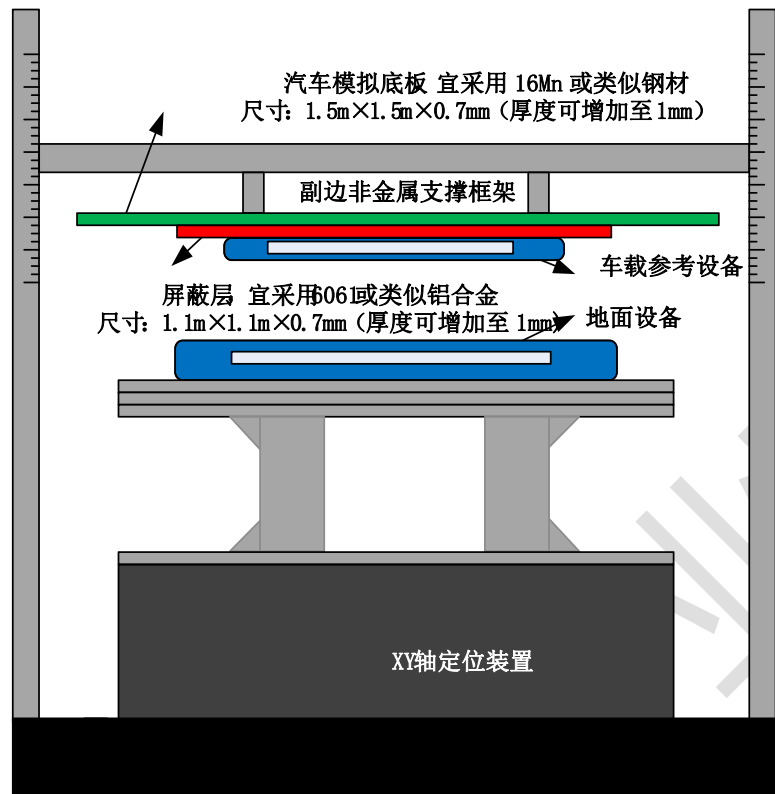
图 5 部件级测试
