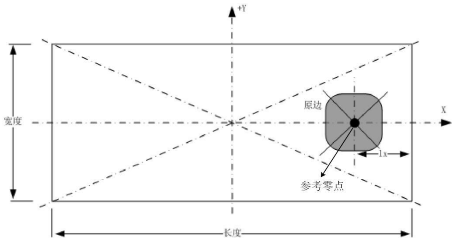
图 2 原边设备的安装位置
