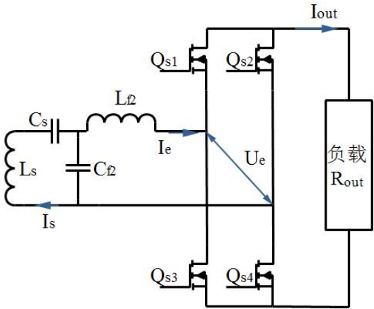
图 B.12 MF-WPT3 车载参考设备的主电路拓扑
