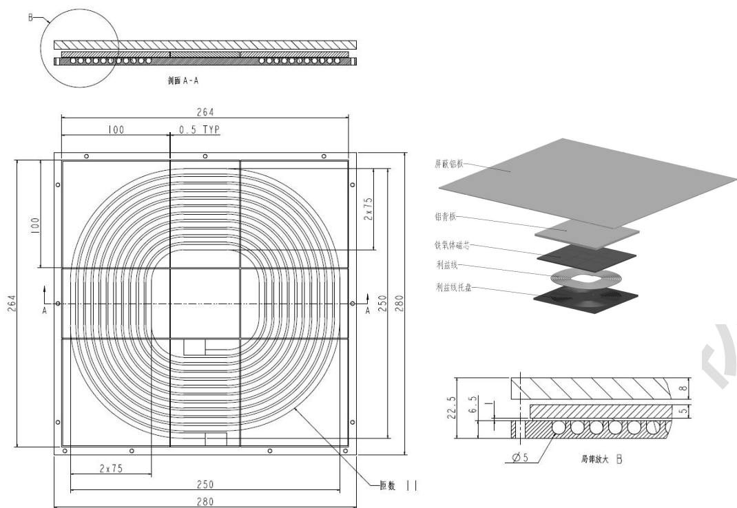
图 B.5 MF-WPT2 Z1 的车载参考设备的机械结构
