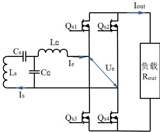
图 B.4 MF-WPT1 车载参考设备的主电路拓扑
