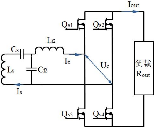
图 B.8 MF-WPT2 车载参考设备的主电路拓扑
