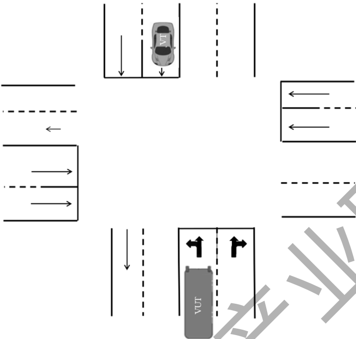
图10 左转车辆冲突通行试验场景示意图
