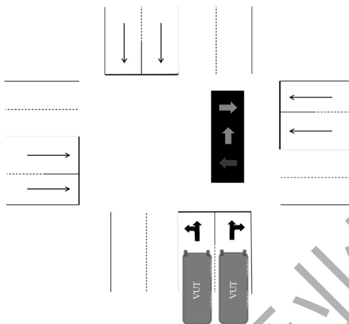
图5 方向指示信号灯试验场景示意图
