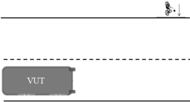
图16 自行车横穿道路试验场景示意图
