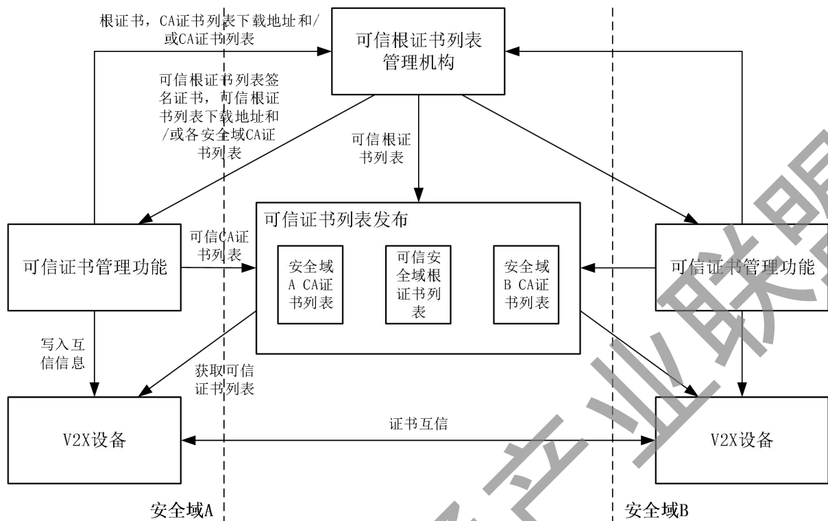
图 5 PKI 互信架构
