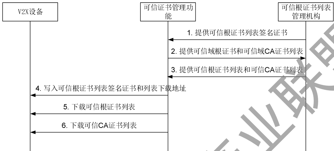
图 7 集中式 PKI 互信管理的一般过程
